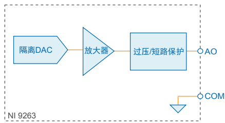
图 1. NI 9263 某通道的输出电路
